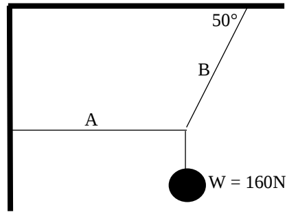
Diagrama de cuerpo libre
