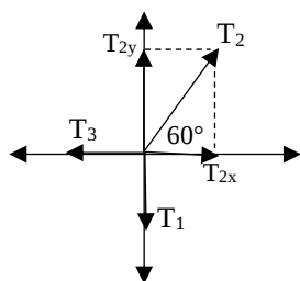
Diagrama de cuerpo libre
